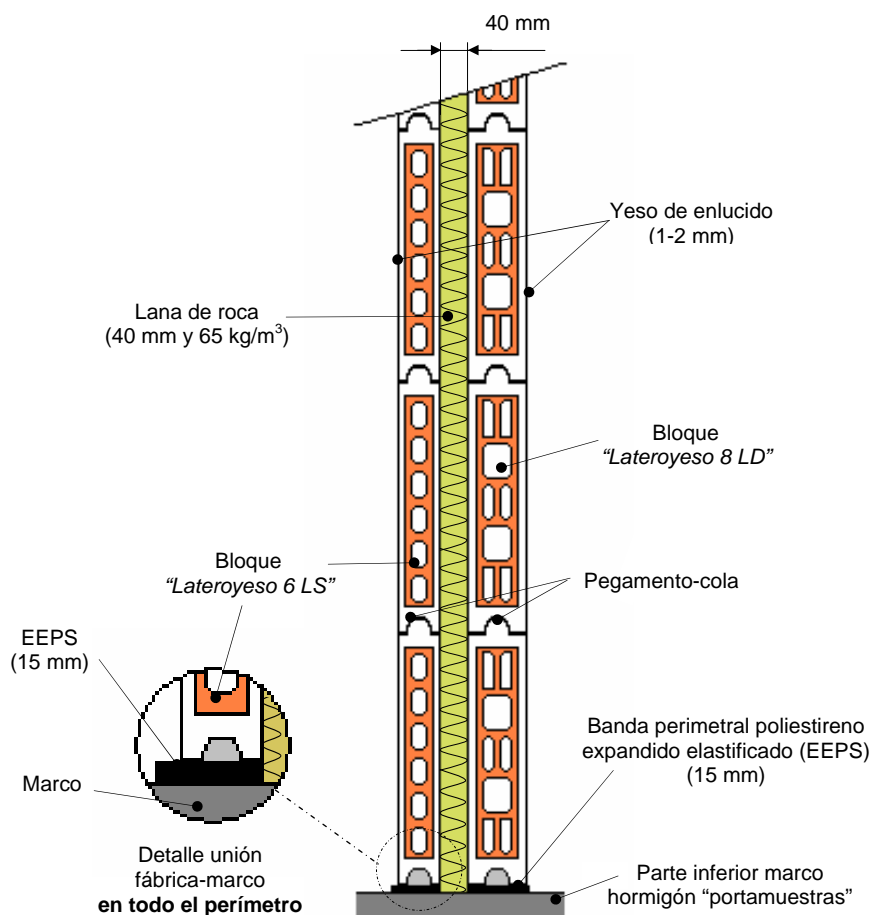
Figura 1: Esquema de la muestra ensayada (B0812-39-M71)
