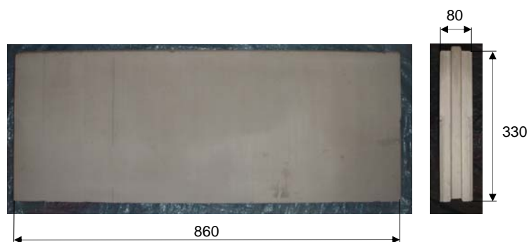
Figura 3: Dimensiones del bloque “Lateroyeso 8 LD” (Cotas en mm)
