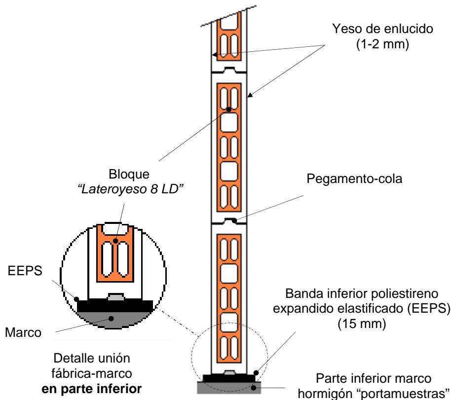
Figura 1: Esquema de muestra ensayada (B0910-04-M03)
