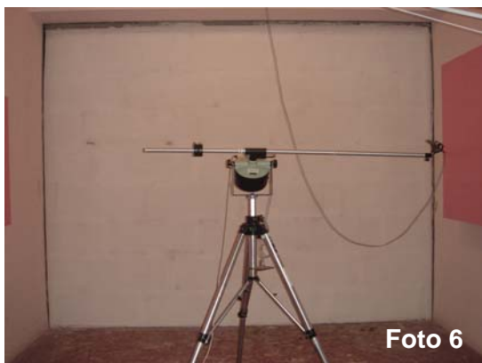
Fotos 6 y 7: Vistas de muestra en cámaras de ensayo
