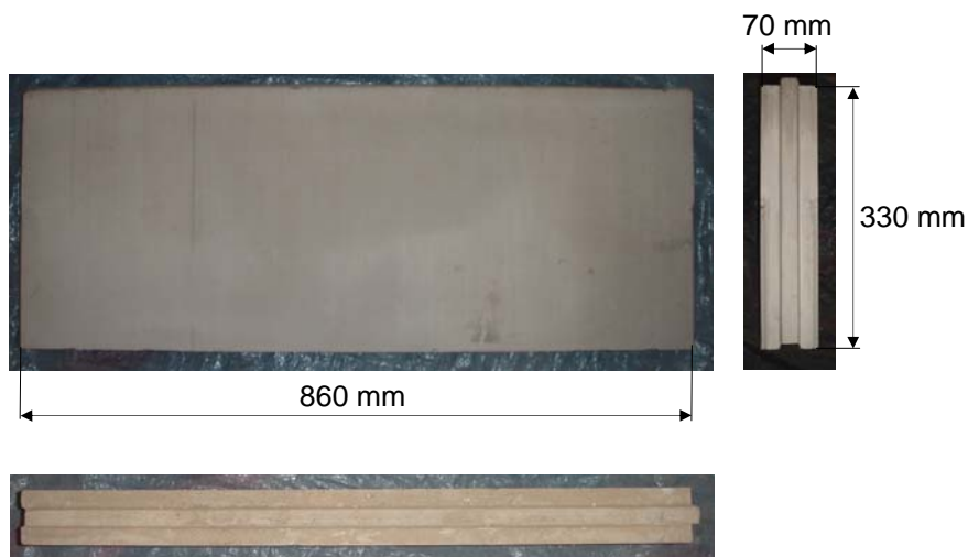
Figura 3: Dimensiones de bloque “Lateroyeso 7 LD”
