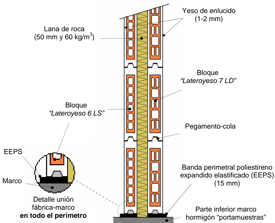
Figura 1: Esquema de la muestra ensayada (B0160-07-HILAY-02-M284)
